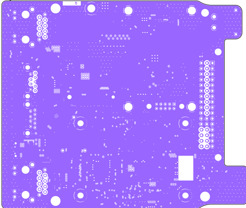
Layer 5 (Scale 1:1)
