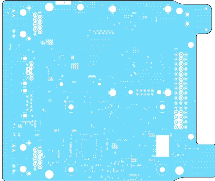
Layer 4 (Scale 1:1)
