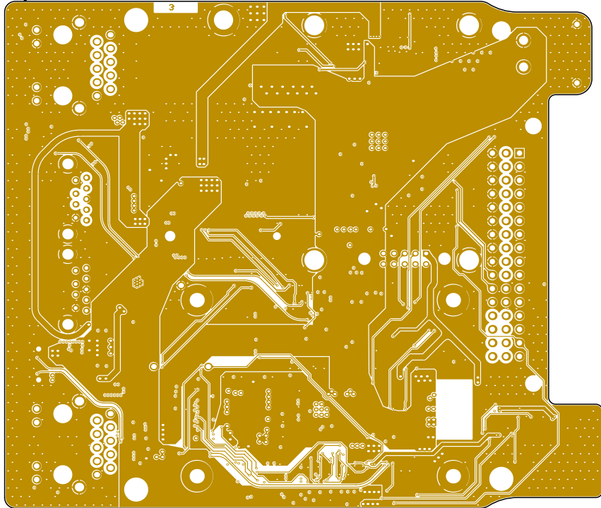
Layer 3 (Scale 1:1)
